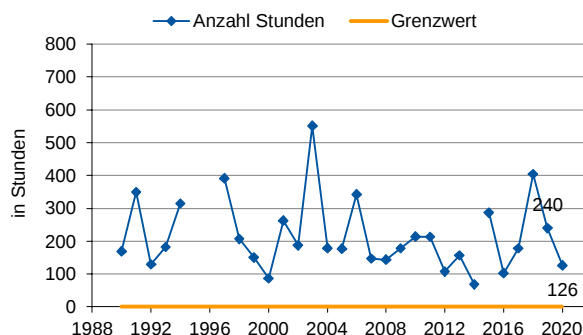
Ozon-Konzentration
